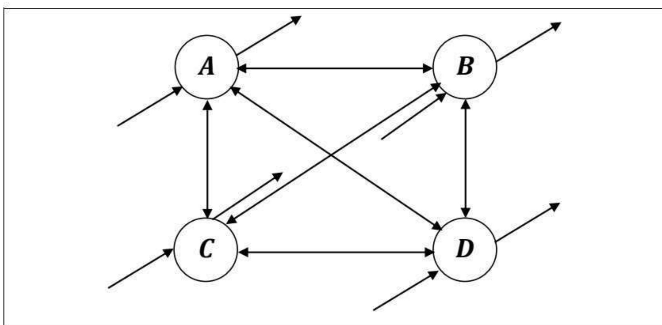
Figure 3.8 : Réseau de Hopfield à 4 neurones.
