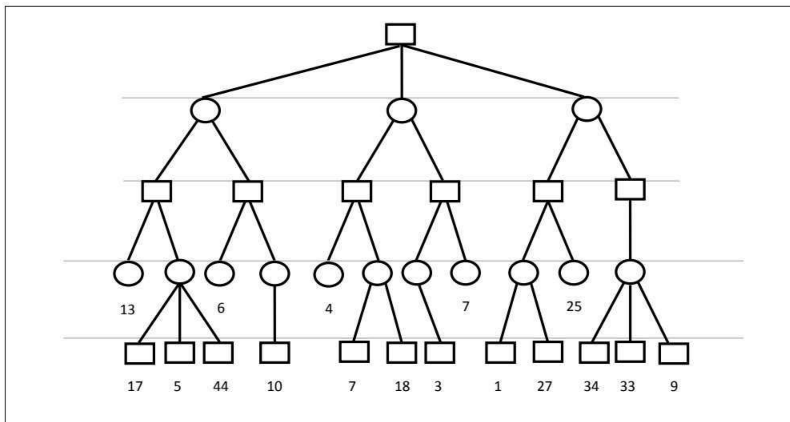
Figure 1.7 : Exemple d'arbre de jeu.
