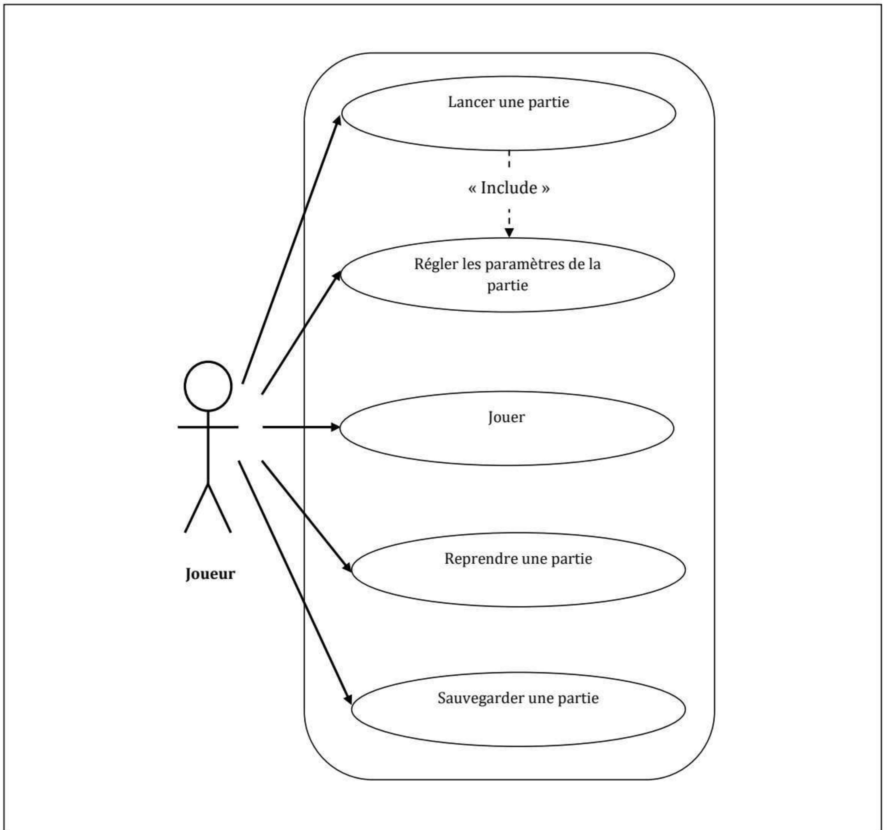
Figure 4.12 : Diagramme de cas d'utilisation « Joueur».
