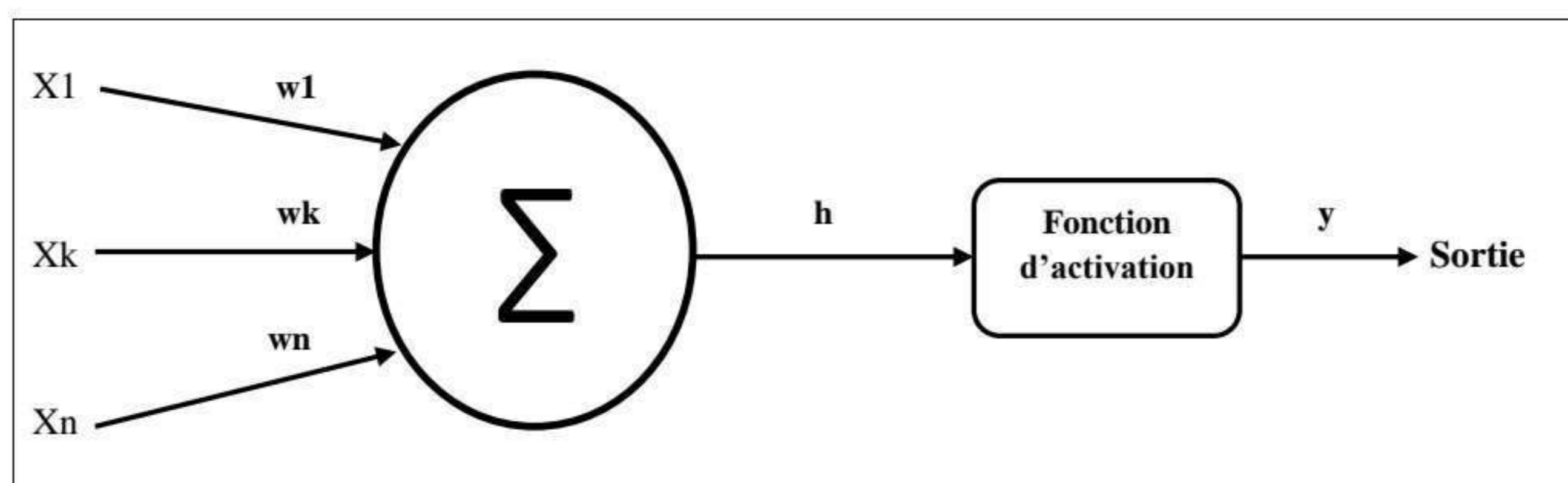
Figure 3.3: Neurone formel mathématique.
