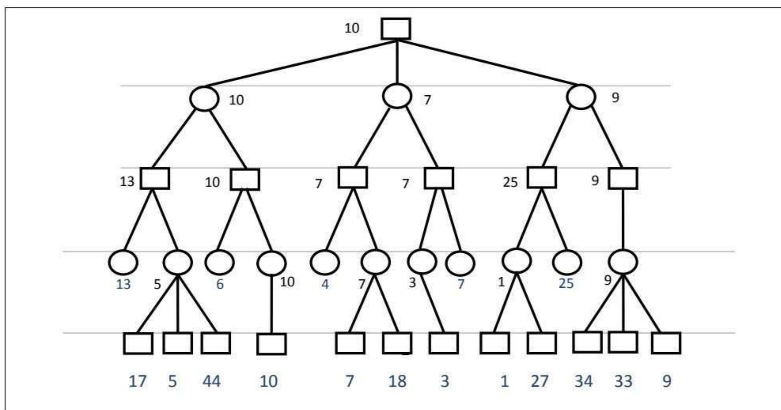
Figure 1.8 : Exemple résolu avec l'algorithme du Minimax.
