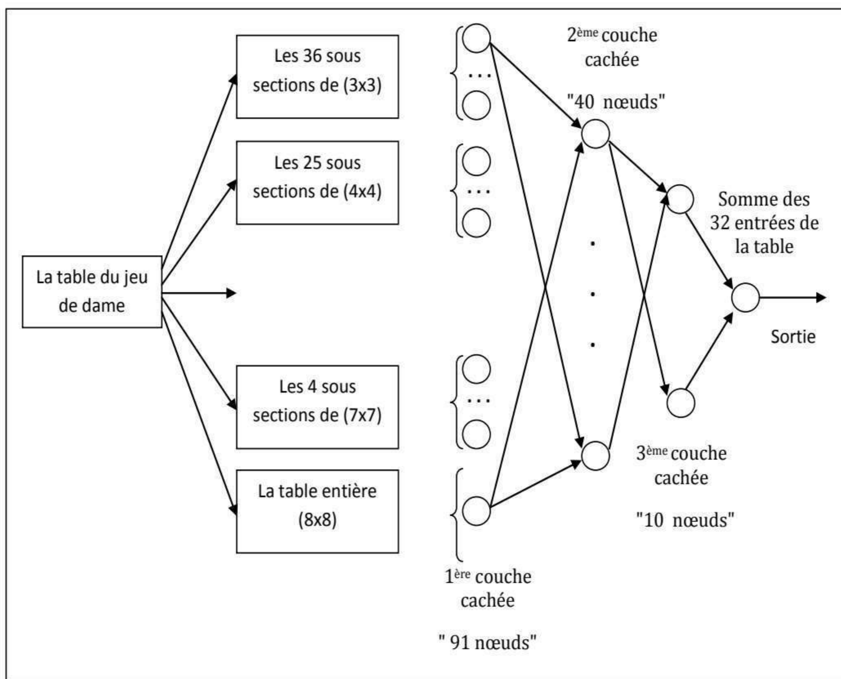
Figure 4.6 : Structure du réseau de neurones
