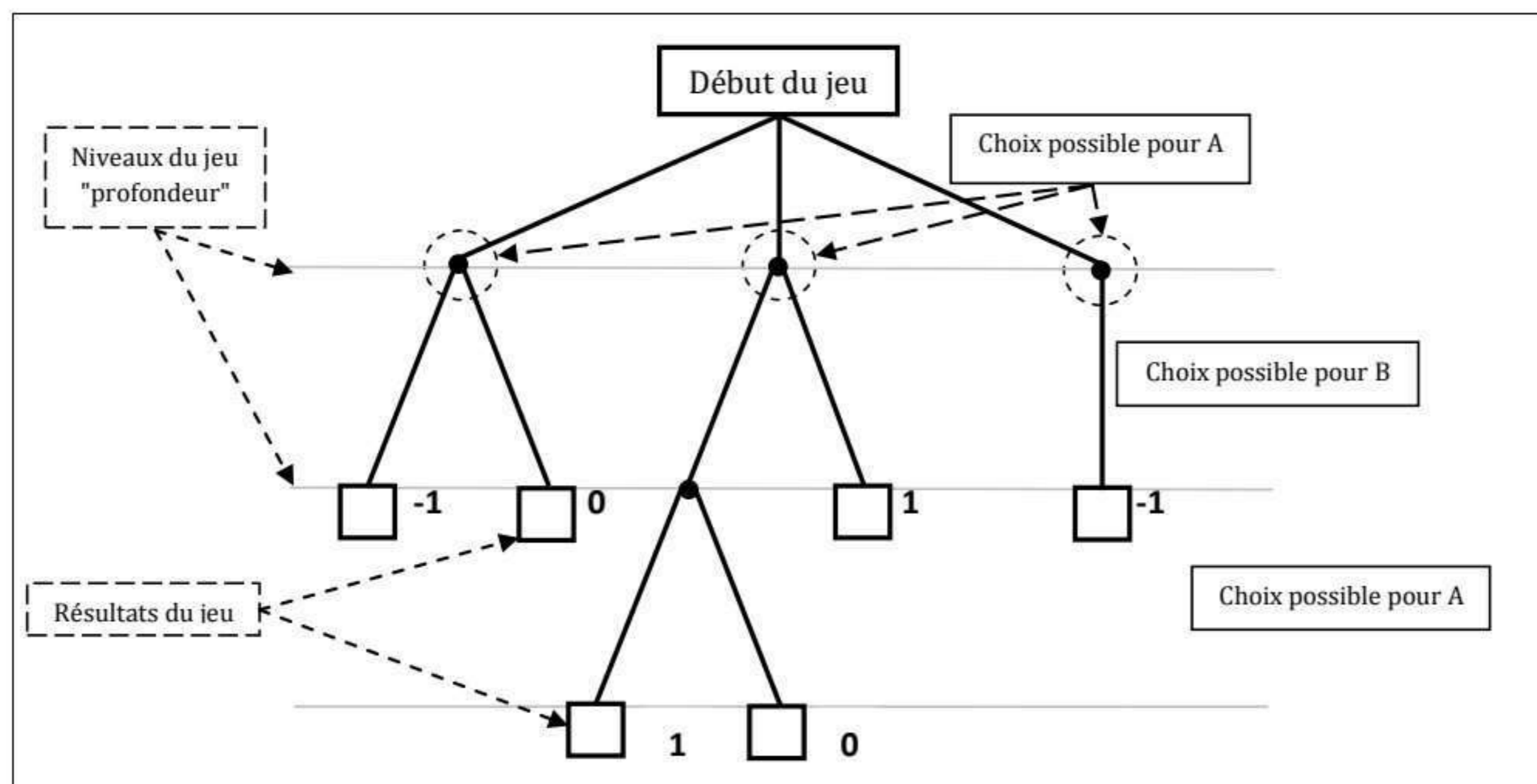
Figure 1.2 : Exemple de représentation arborescente d'un jeu.
