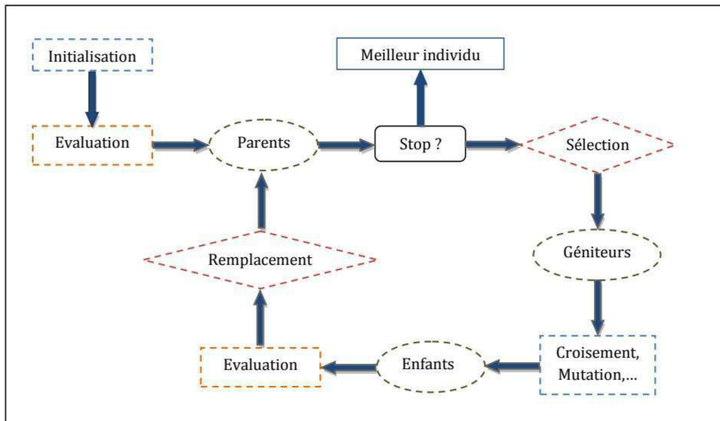
Figure 2.2: Organigramme d'un algorithme évolutionnaire.
