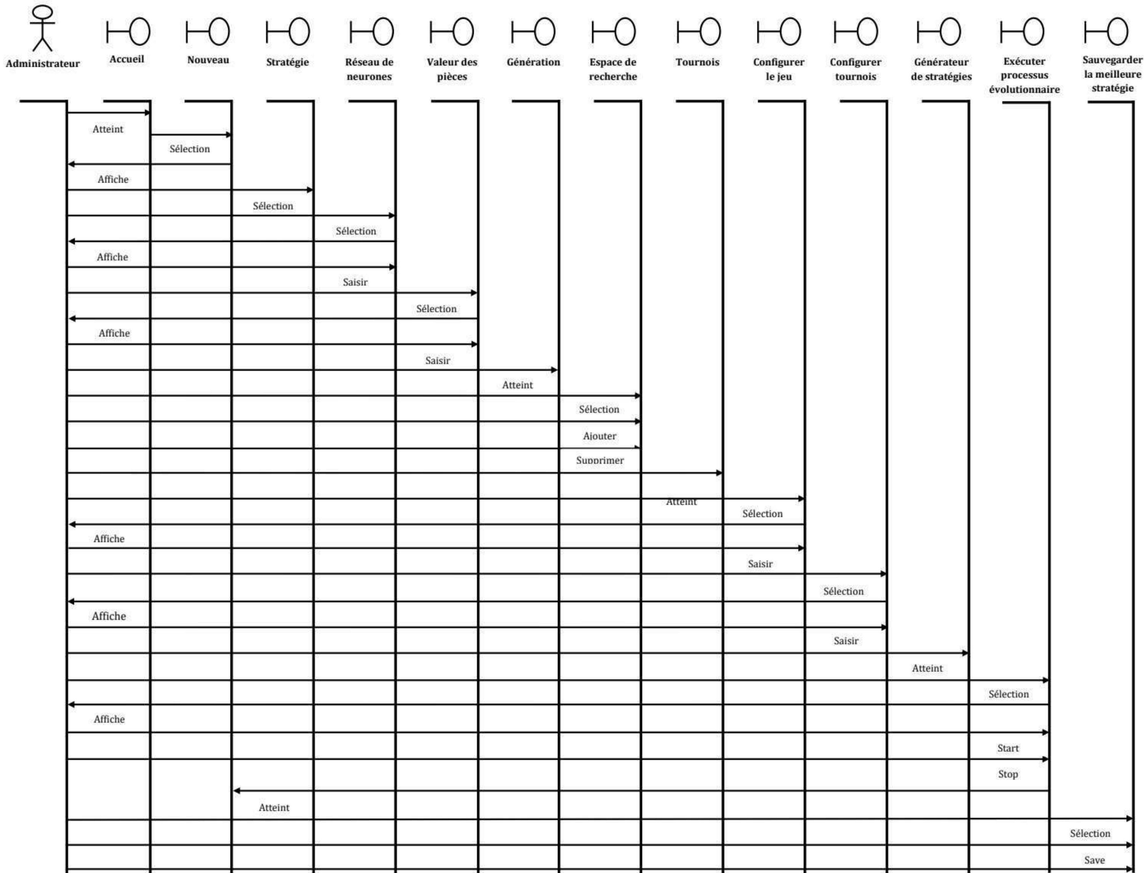
Figure 4.14 : Diagramme de séquence « Créer une Stratégie ».
