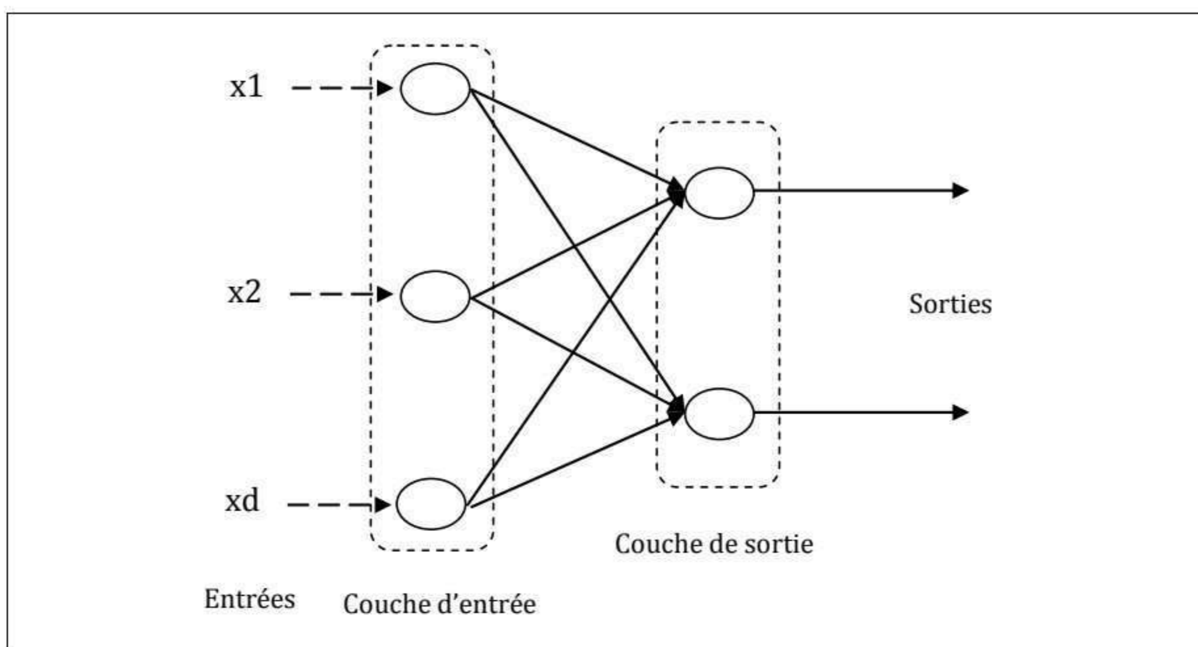
Figure 3.5: Schéma d'un perceptron mono-couche.
