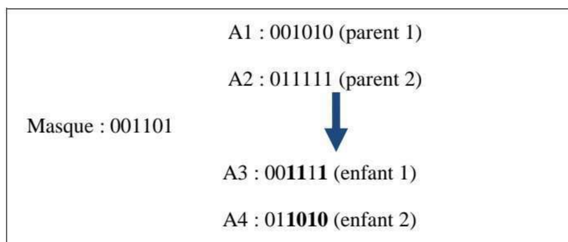
Figure 2.4 : Croisement uniforme.
