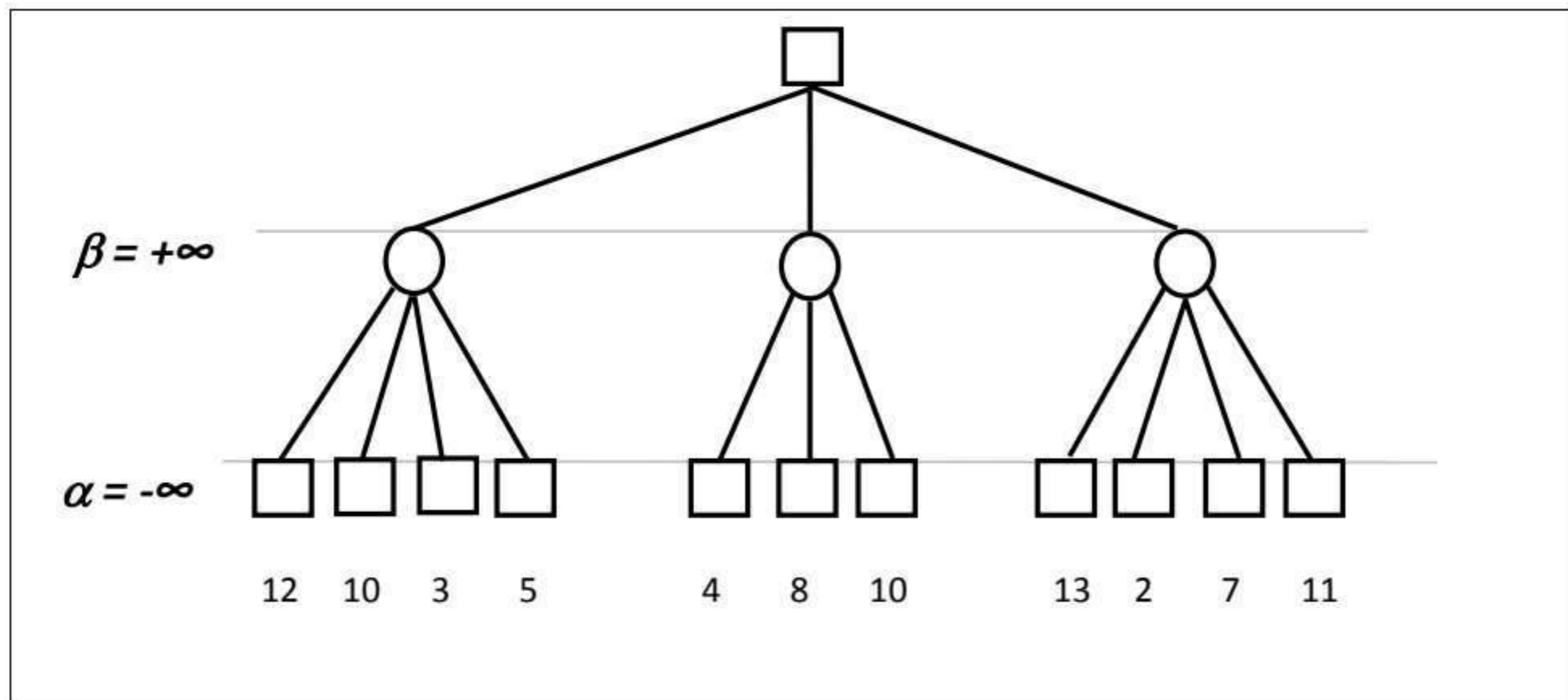
Figure 1.9 : Exemple d'arbre de jeu.
