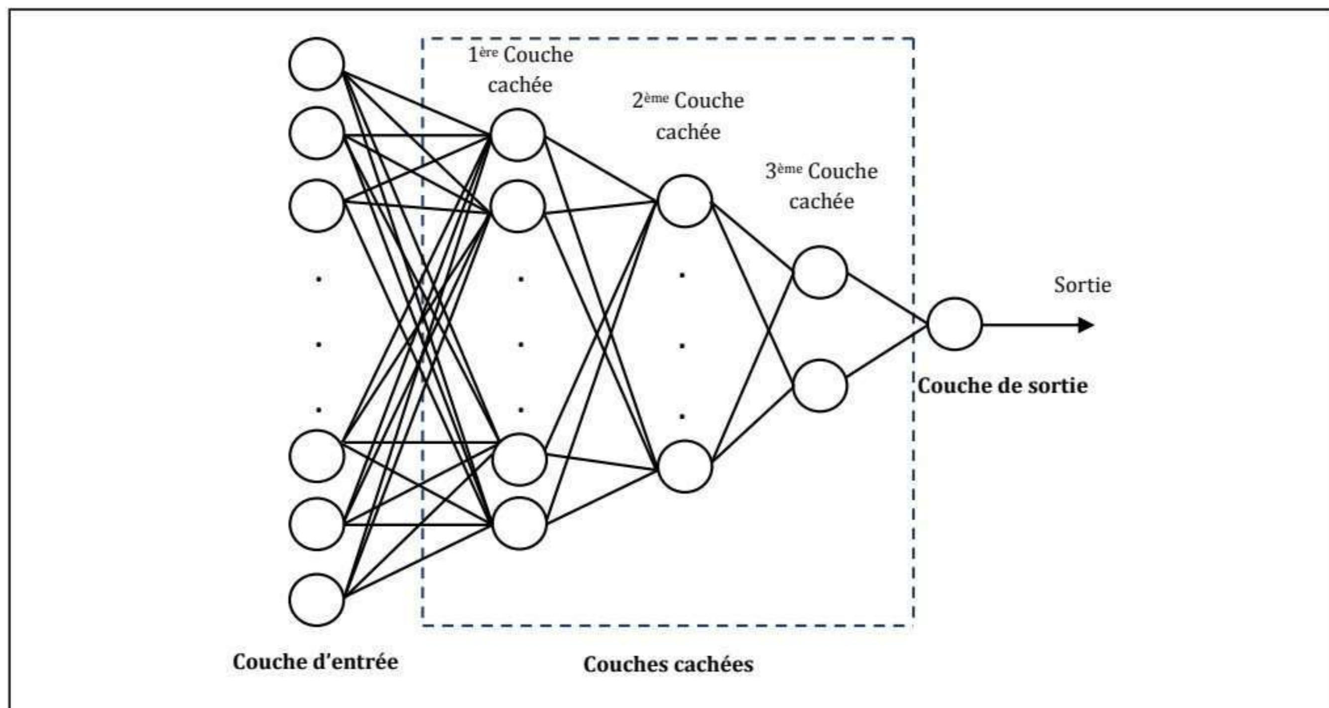
Figure 4.5 : Architecture du Réseau de neurones.
