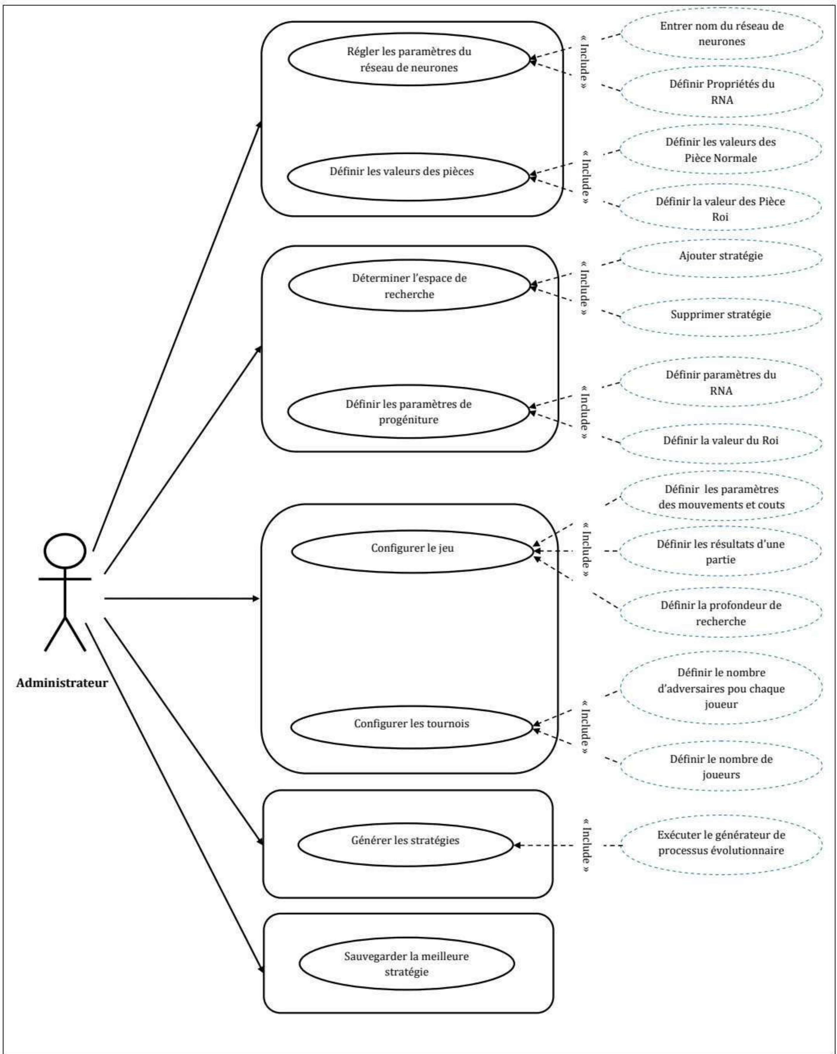
Figure 4.11 : Diagramme de cas d'utilisation « Administrateur ».
