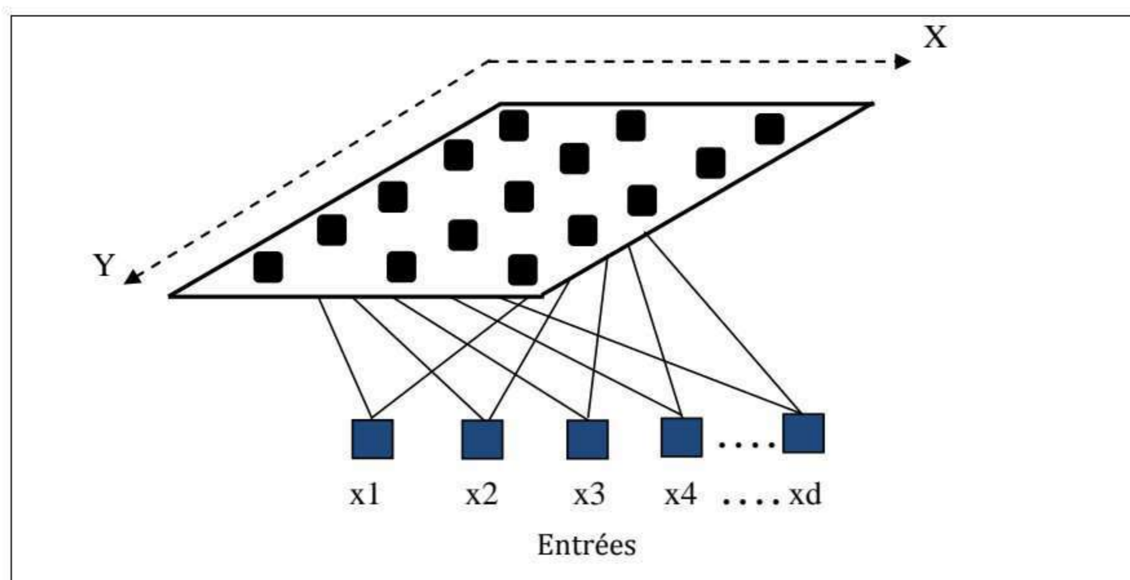
Figure 3.7: carte auto-organisatrice à deux dimensions.
