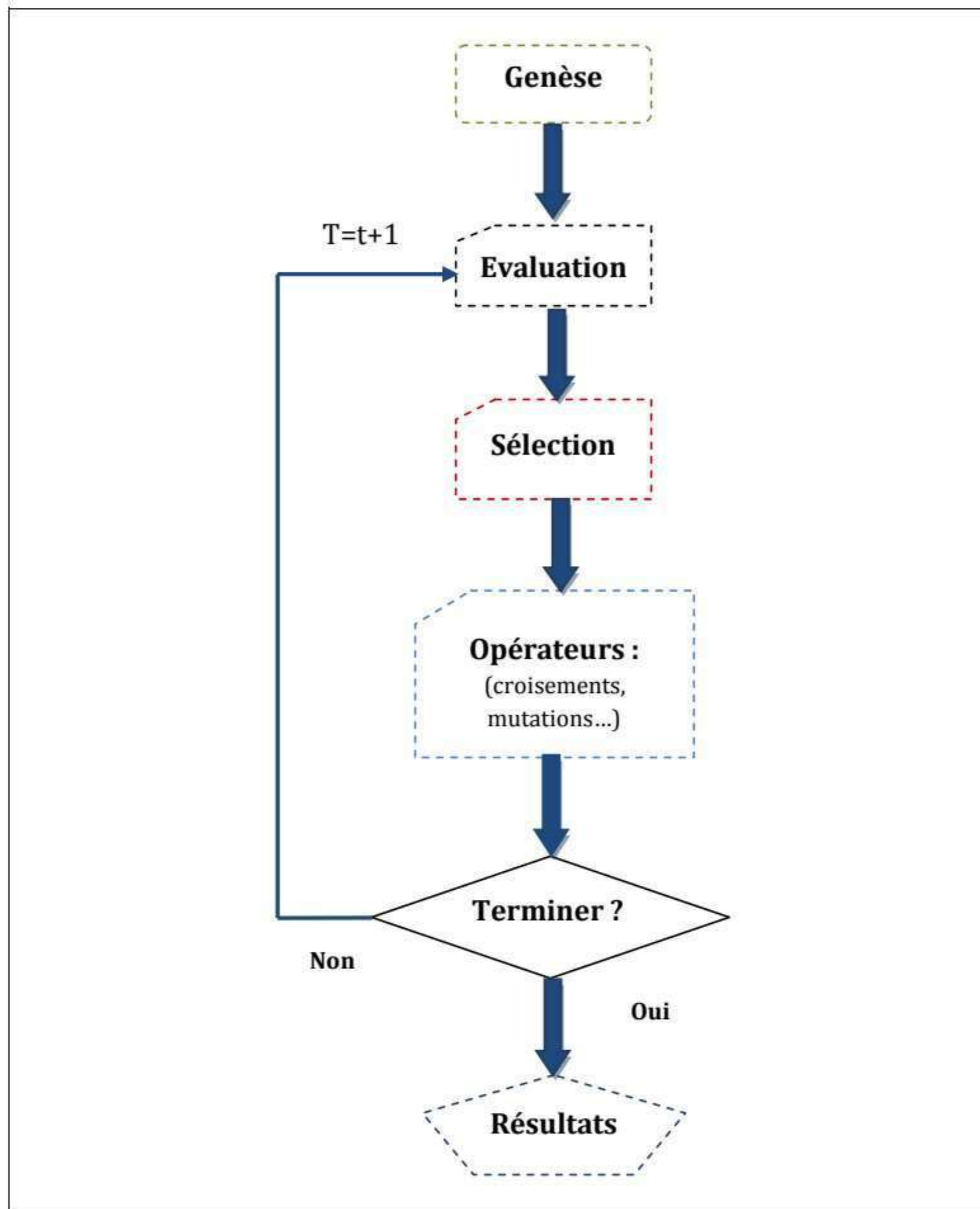
Figure 2.7: Organigramme d'un algorithme génétique.
