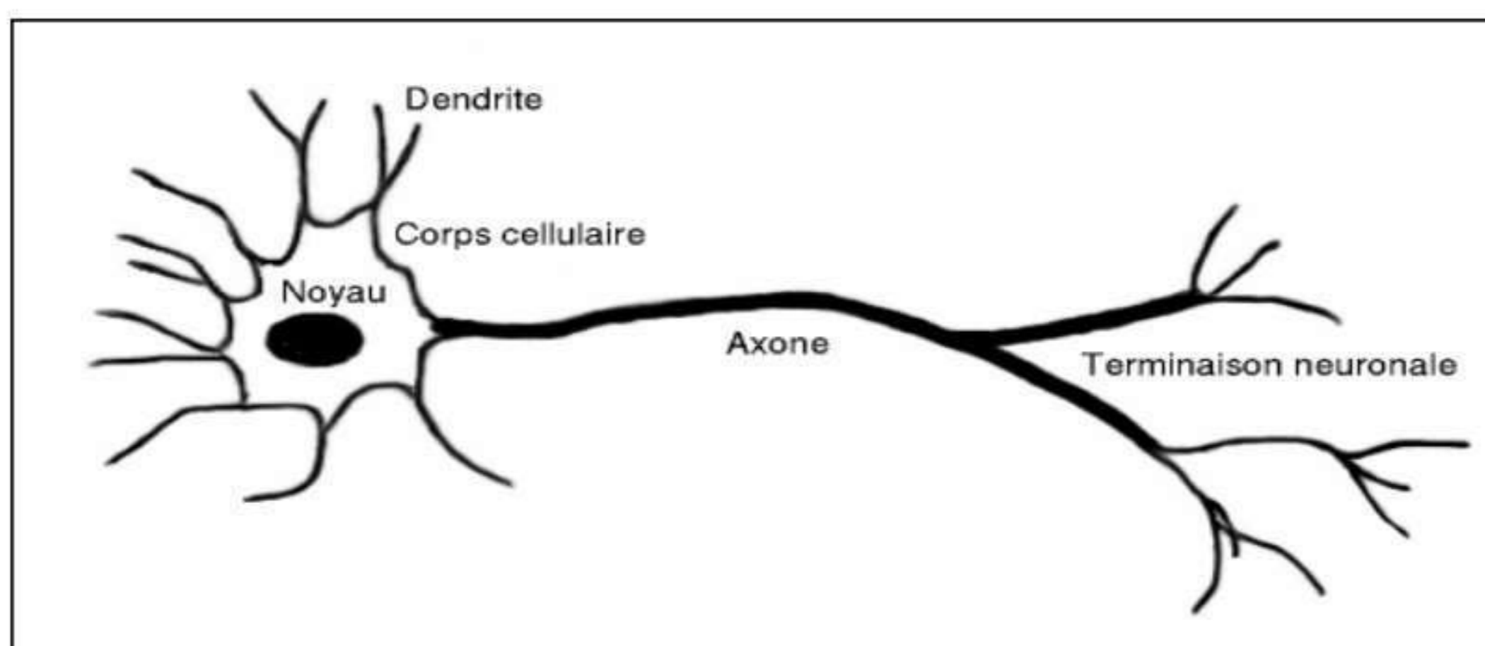
Figure 3.1: Neurone biologique.
