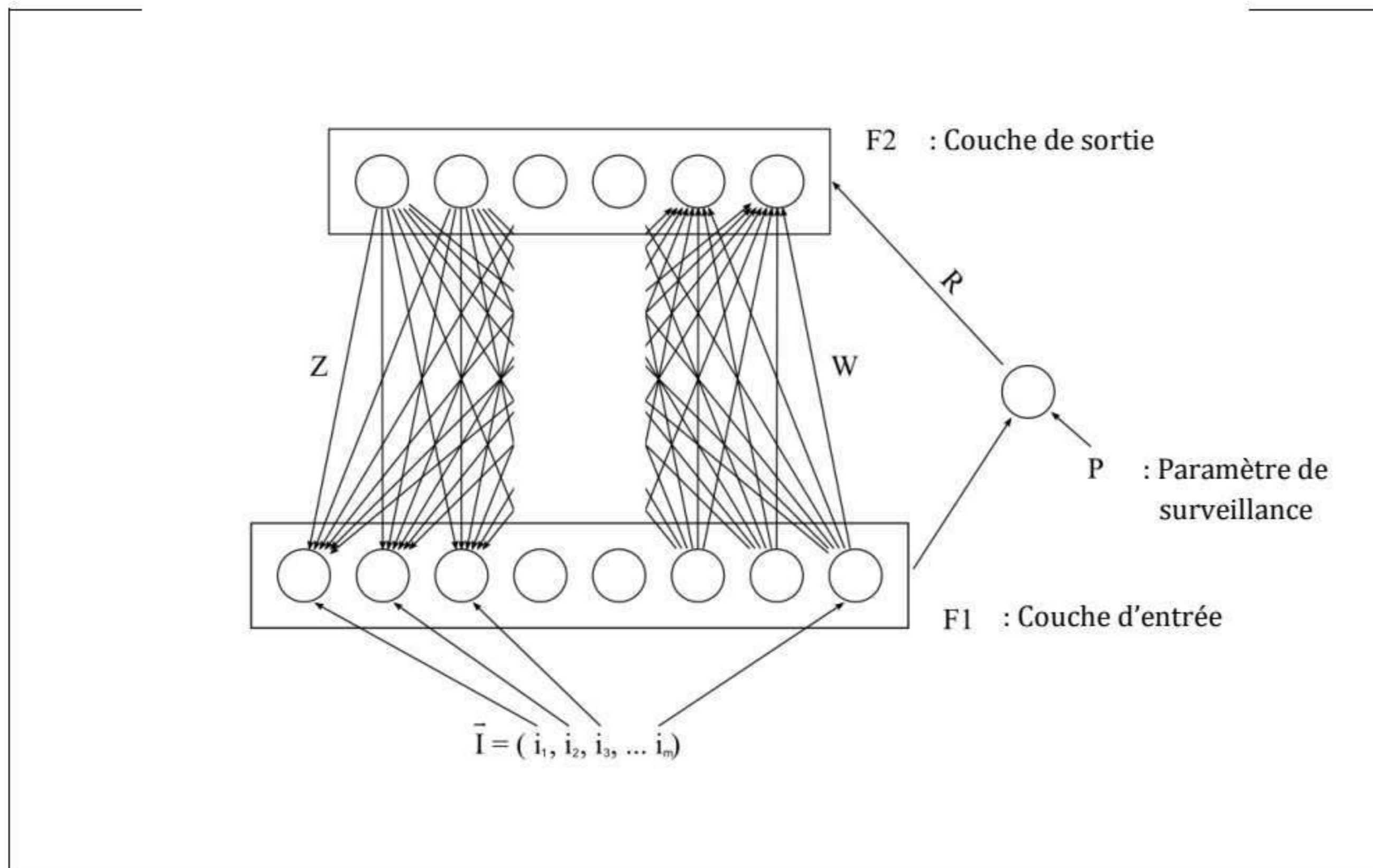
Figure 3.9: Réseau ART.
