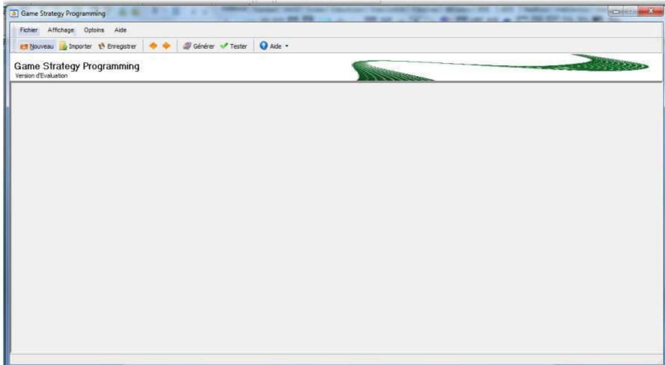
Figure 5.1 : Interface d'accueil.
