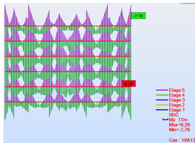
Figure V.9 : Moment diagrams flexing My to the ALS
