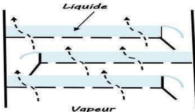
Figure II. 1 : Plateaux perforés. [12]
