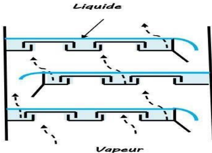
Figure II. 2 : plateaux à calottes [13]
