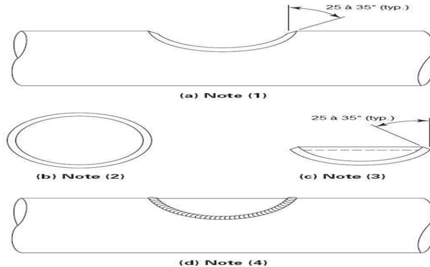
Figure IV. 9 : Type d'insertion d'une plaque soudée dans un tube
