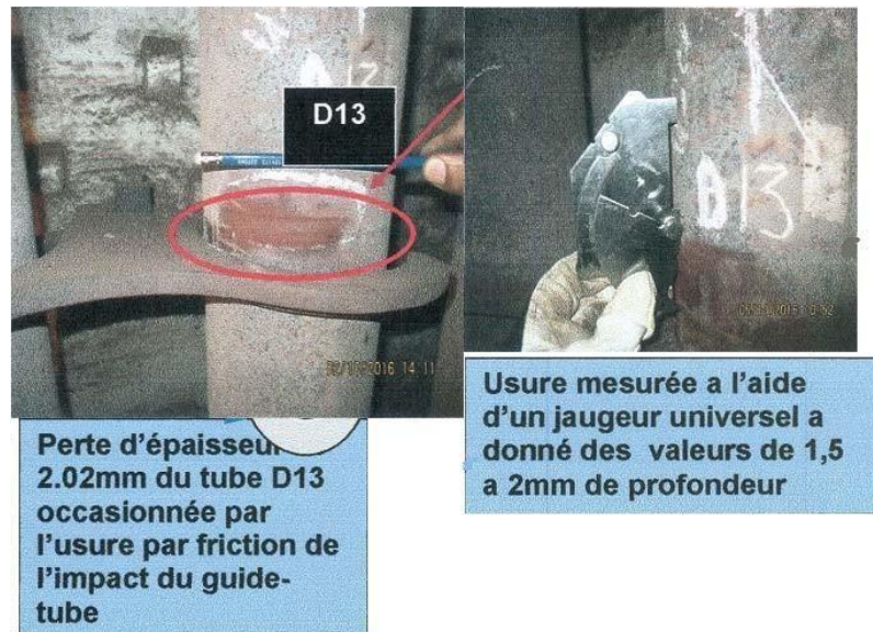
Figure IV. 4 : Usure des tubes par friction en 2016, Four 100-F-102 [44]
