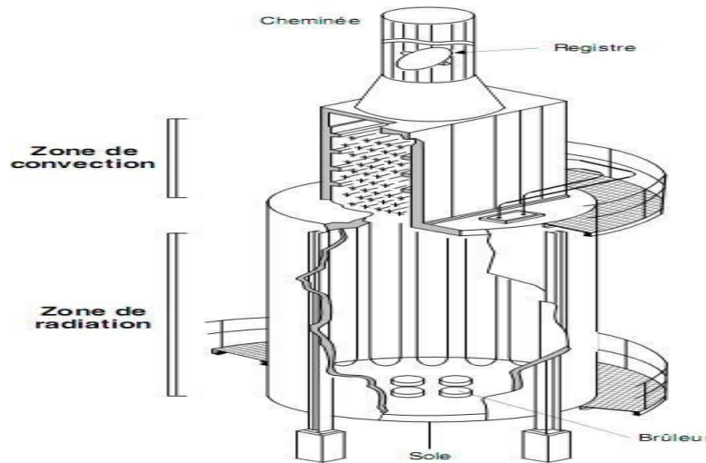
Figure II.9 : Coupe d'un four cylindrique vertical [24]
