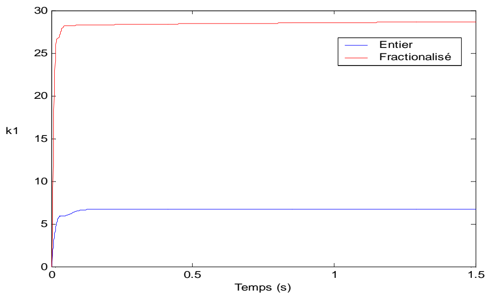
Figure.IV.14.Evolution de paramètre k_1 .
