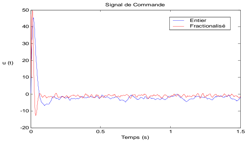
Figure.IV.13.Les signaux de commande d'unPI Adaptatif entier et fractionalisé ( \alpha=0.3 ).
