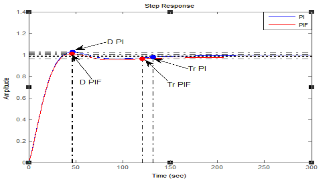
Figure IV.7 : Commande PI et PI fractionalisée d'un radiateur.
