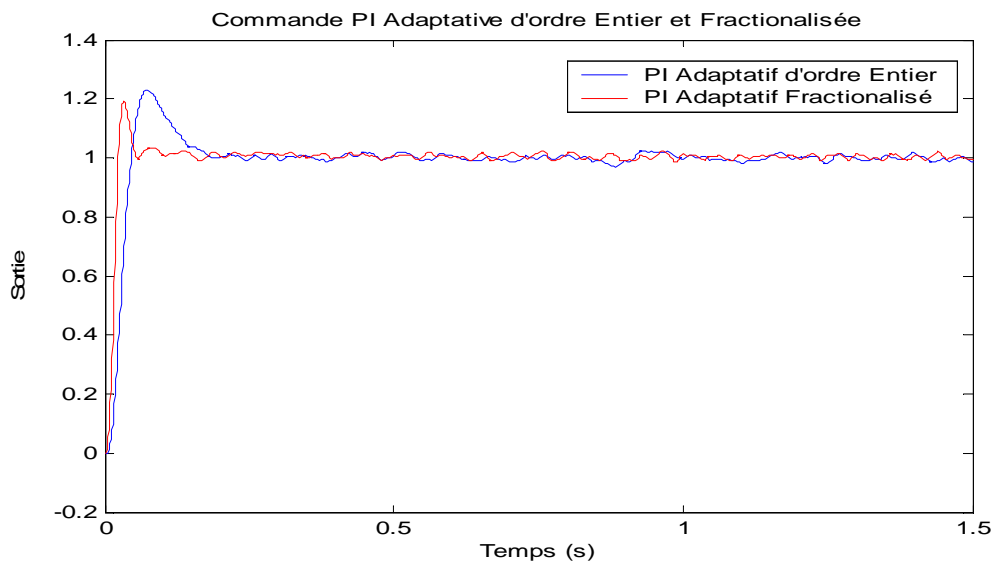
Figure IV.12. Sortie du MCC après l'application de la commande PI adaptative entier et fractionnée ( \alpha=0.3 ) avec bruit aléatoire à la sortie (amplitude 5% du signal de référence)
