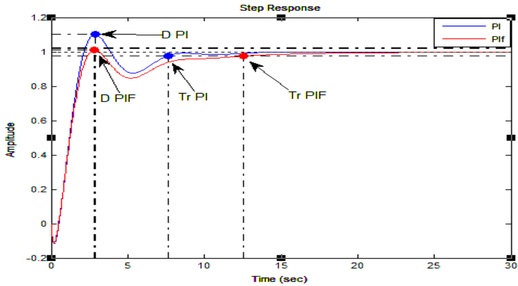
Figure IV.6 : Commande PI et PI Fractionisée d'un système 3 ème ordres
