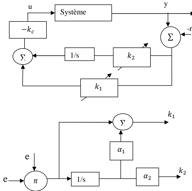
Figure.IV .4. Contrôleur PI adaptatif d'ordre entier.
