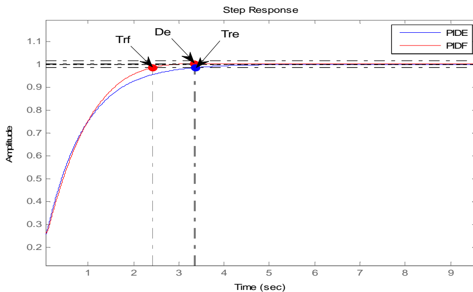
Figure IV.9 : Commande PID et PID fractionalisée d'un Mcc.
