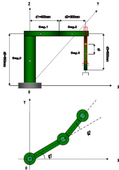
Figure II.6: Schéma du robot SCARA à 3 d.d.l
