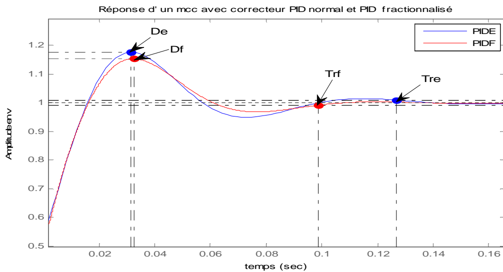
Figure IV.11. Commande PID et PID fractionnée d'un modèle de 2 ème ordre.
