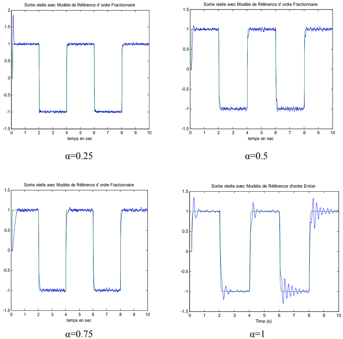
Figure. II.19: Sortie de la Cammande Adaptative à modèle de référence d'ordre fractionnaire pour \alpha=0.25 , \alpha=0.5 , \alpha=0.75 , \alpha=1 avec bruit aléatoire à la sortie(amplitude 5% du signal de référence)
