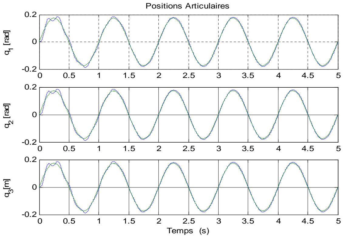
Figure II.11. La position articulaire du robot et la trajectoire de référence en utilisant la commande MRAC d'ordre Fractionnaire ( \alpha=0.3 )
