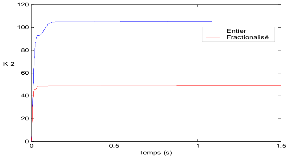
Figure.IV.15.Evolution de paramètre k2.
