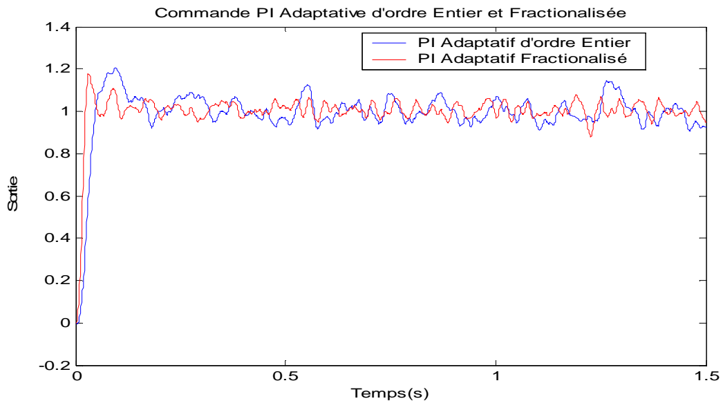
Figure IV.16. Sortie du MCC après l'application de la commande PI adaptative entier et fractionalisée ( \alpha=0.3 ) avec bruit aléatoire à la sortie(amplitude 5% du signal de référence)
