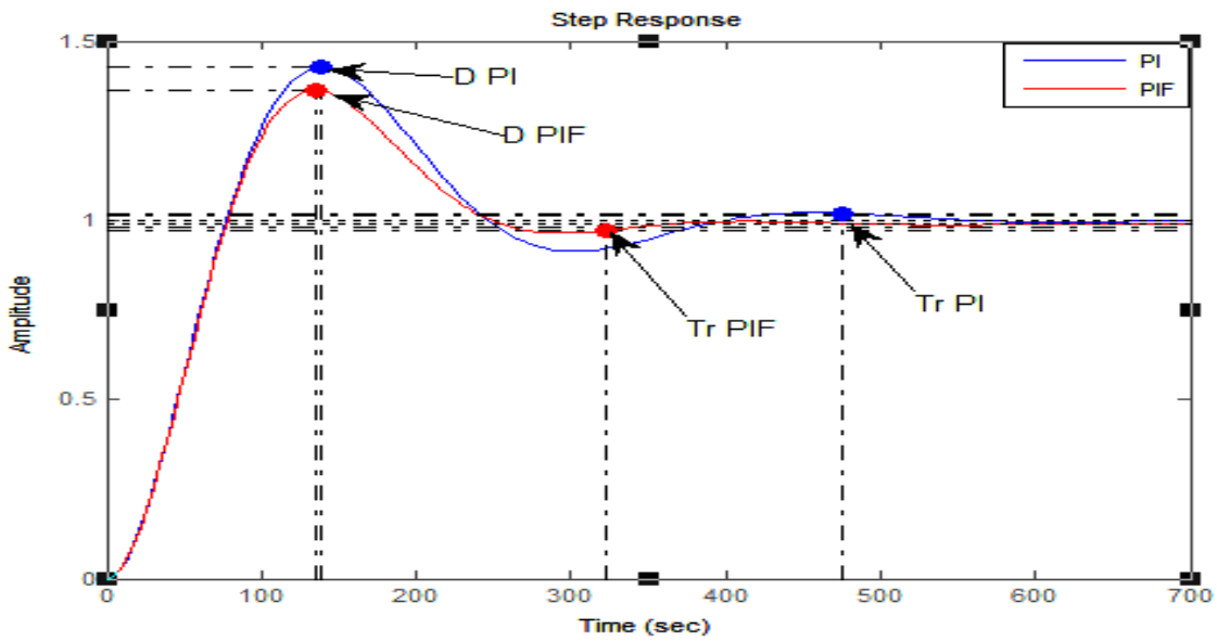
Figure IV.8. Commande PI et PI fractionnisée d'un four.
