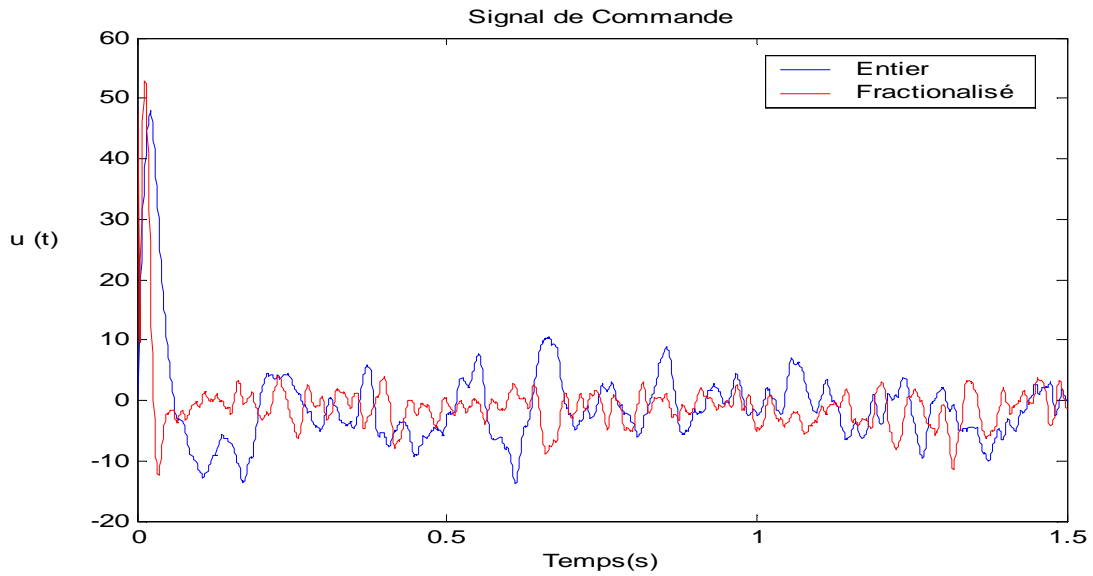
Figure.IV.17.Les signaux de commande de PI adaptatif entier et fractionné( \alpha=0.3 ).
