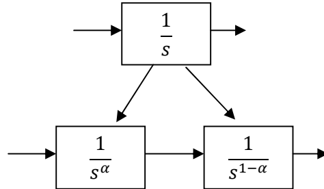
Figure IV .3.Fractionalisation d'un intégrateur
