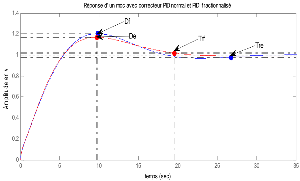
Figure IV.10. Commande PID et PID fractionnée d'un Radiateur.
